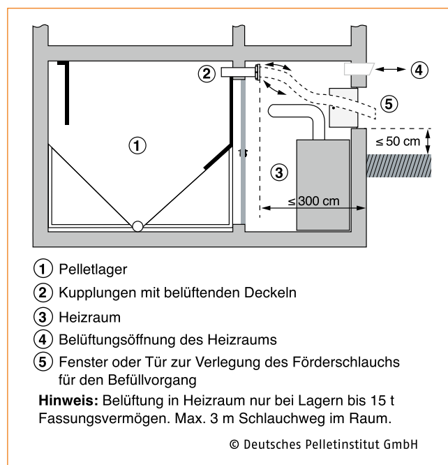
Abb. 31: Belüftungslösung für Pelletlager mit Stutzen im Heizraum (Lüftungskonzept erforderlich)
